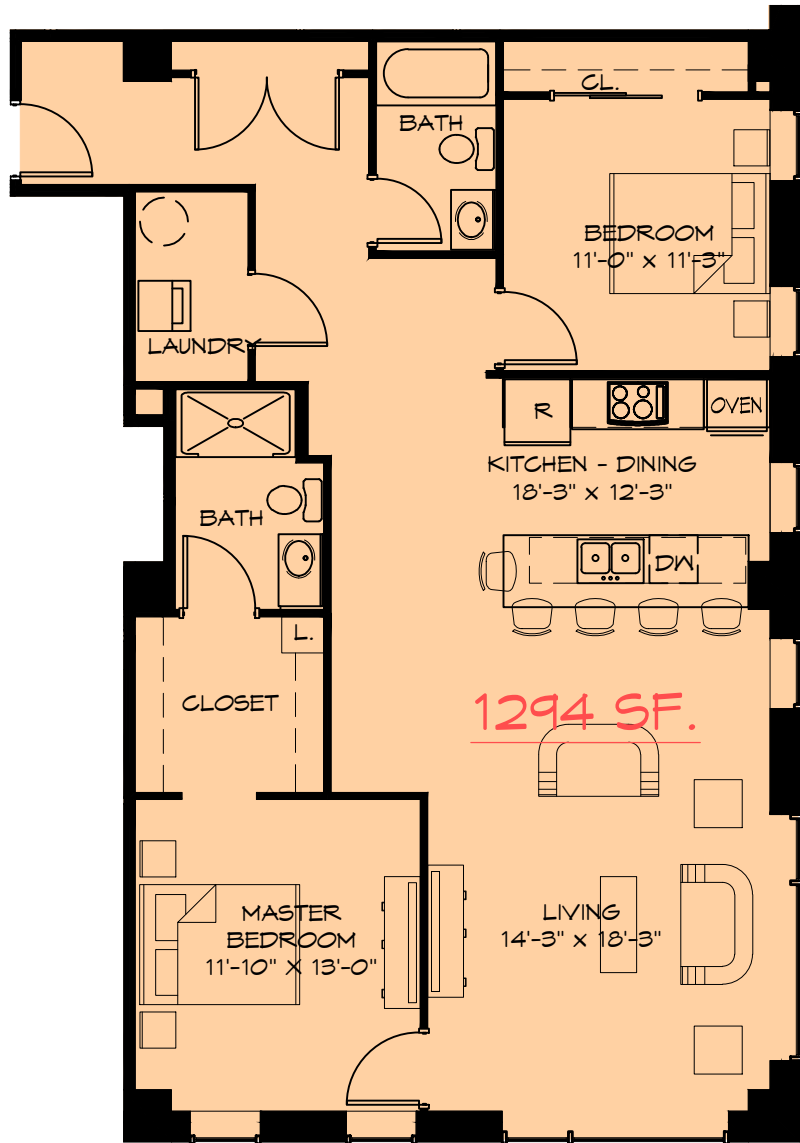
UNIT 3 SCALE: 1/8"=1'-0"
