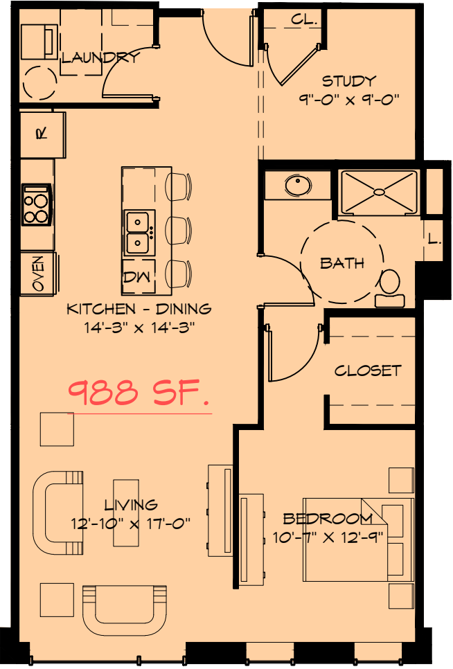
UNIT 4 SCALE: 1/8"=1'-0"
