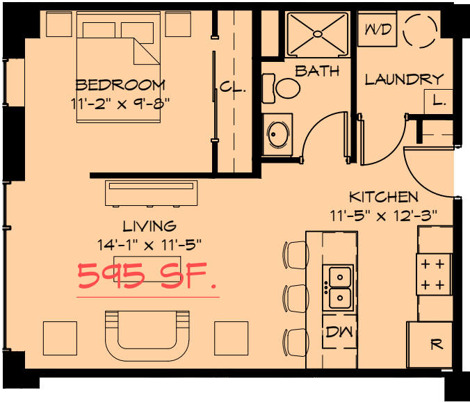
UNIT 8 SCALE: 1/8"=1'-0"
